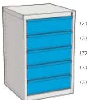
H1000 mm. 5 CASSETTI Art. CL 100 51 estrazione totale
