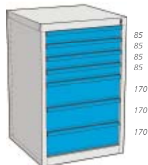
H1000 mm. 7 CASSETTI Art. CL 100 71 estrazione totale
