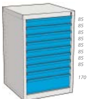
H1000 mm. 9 CASSETTI Art. CL 100 91 estrazione totale
